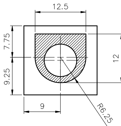
Przekrój A-A (2:1)
